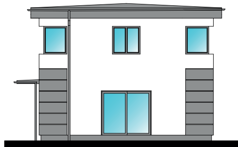
ELEWACJA ZACHODNIA 1:100
