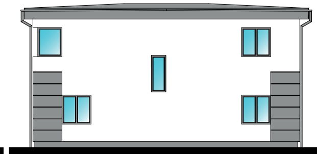
ELEWACJA POŁUDNIOWA 1:100
