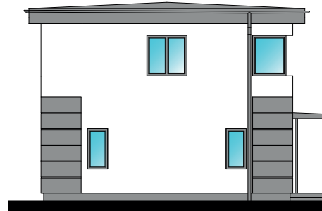
ELEWACJA WSCHODNIA 1:100
