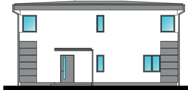
ELEWACJA PÓŁNOCNA 1:100
